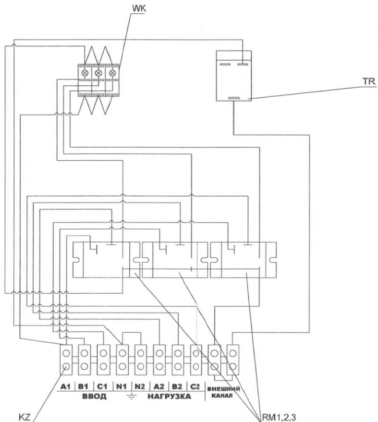
Рис.2 Схема монтажная.
